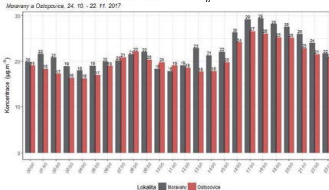
Obr. 3: Průměrný denní chod hodinových koncentrací PM 10
