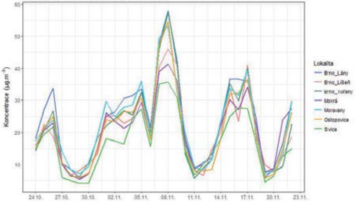
Obř. 4: Vývoj průměrných denních koncentrací PM 10 Výběrná stanice Jihomoravského újeje, 24. 10. - 23. 11. 2017
