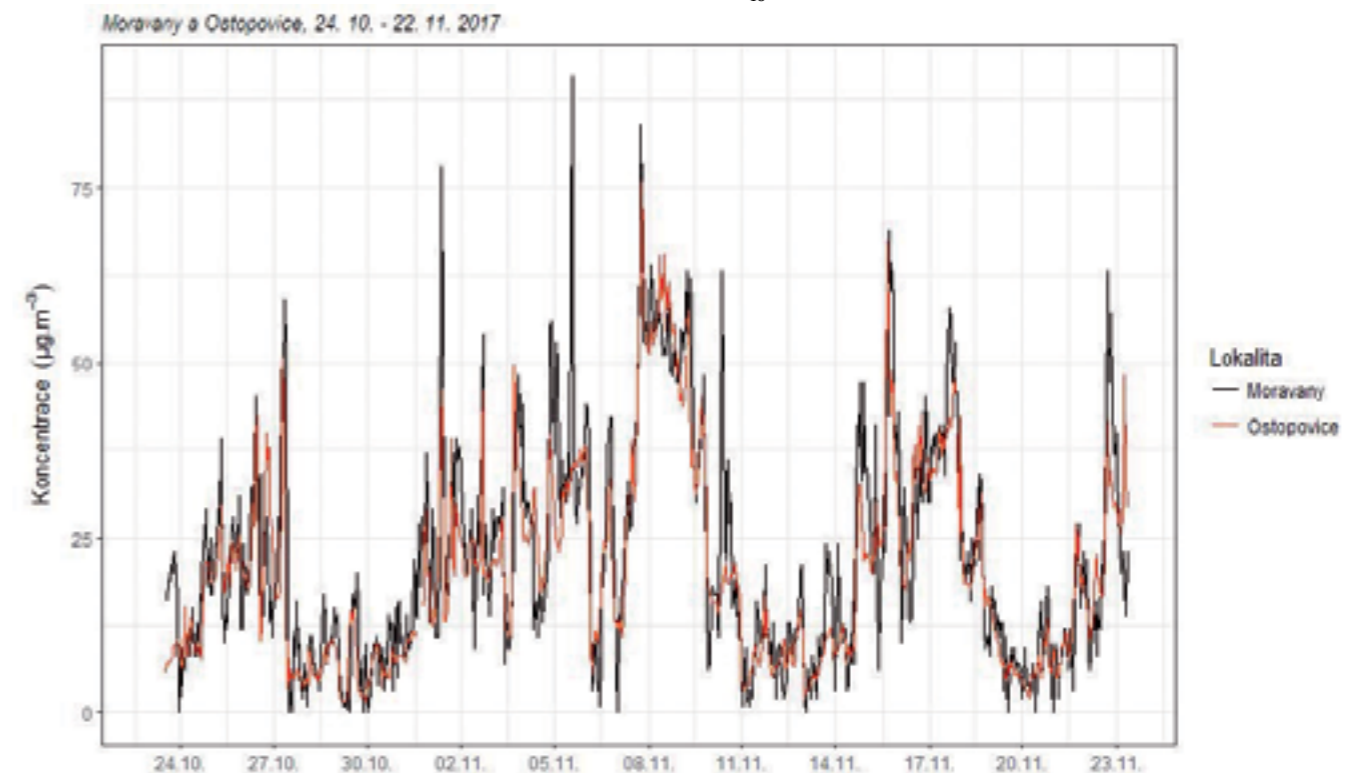
Obr. 1: Vývoj průměrných hodinových koncentrací PM 10
